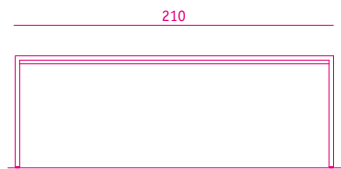
210 x 105 x 74 mit edelstahltraverse
